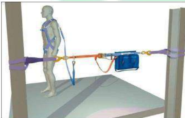
Gbr: Instalasi perangkat penahan jatuh tidak permanen perorangan horizontal (temporary horizontal life mbar dline)
