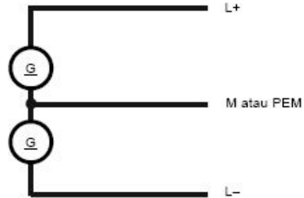
Gambar 7 – 3-kawat
