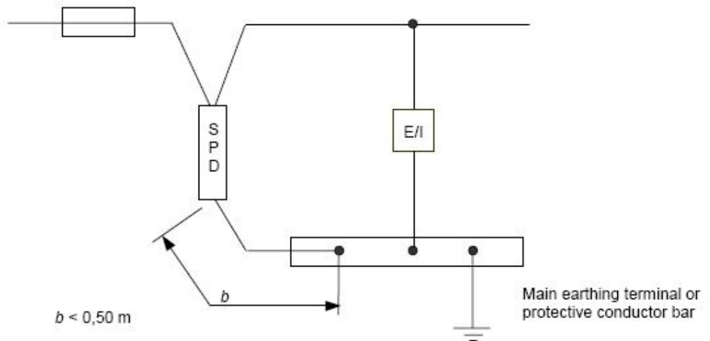
Gambar 53E Contoh pemasangan GPS pada atau di dekat awal instalasi
