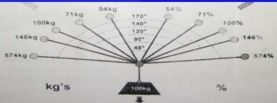
Diagram beban pada penggunaan 2 (dua) akibat sudut angkur
